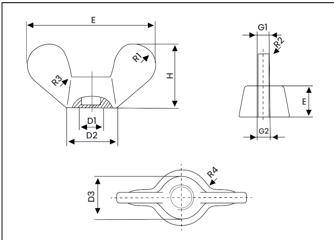
Metric Dimensions – DIN 315 Wing Nut
