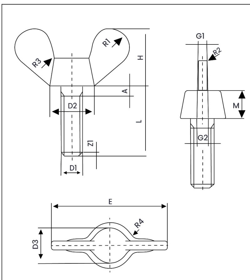
Metric Dimensions – DIN 316 Wing Screw
