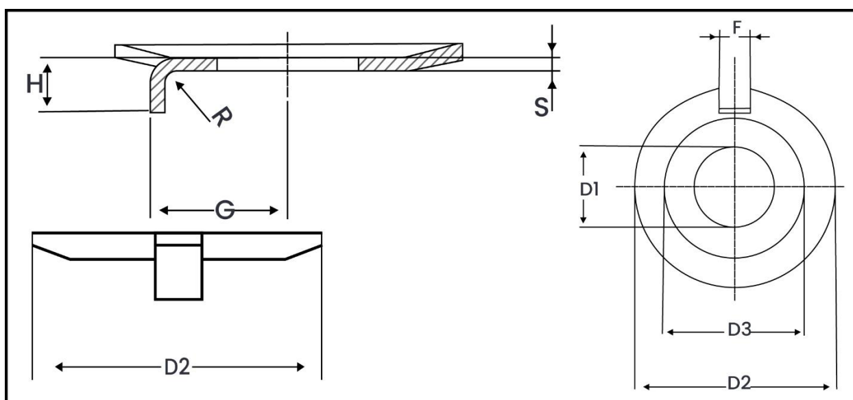
Metric Dimensions – DIN 432 External Tab Washer
