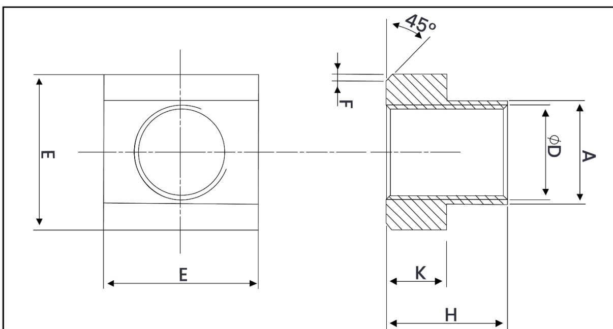
Metric Dimensions – DIN 508 T-Slot Nut
