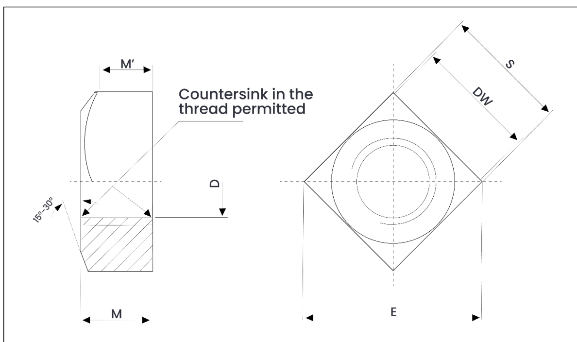
Metric Dimensions – DIN 557 Square Nut
