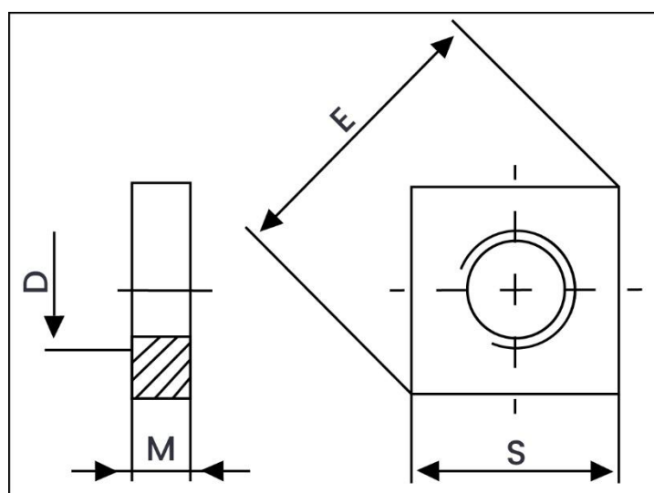
Metric Dimensions – DIN 562 Thin Square Nut
