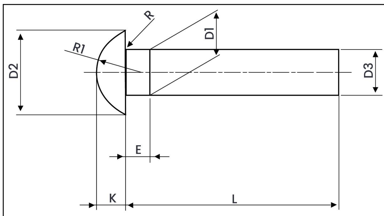
Metric Dimensions – DIN 660 Round Head Rivet
