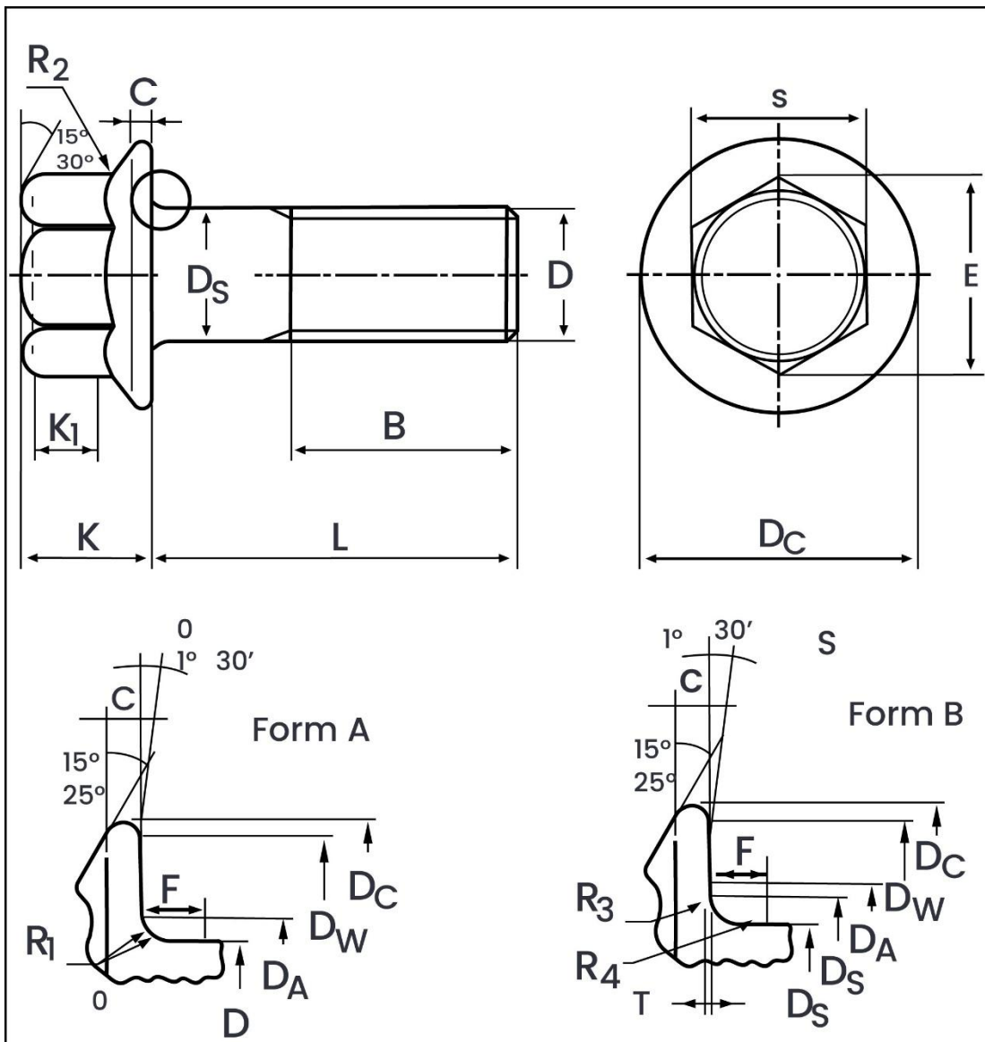
Metric Dimensions – DIN 6921 Hexagon Flange Bolt
