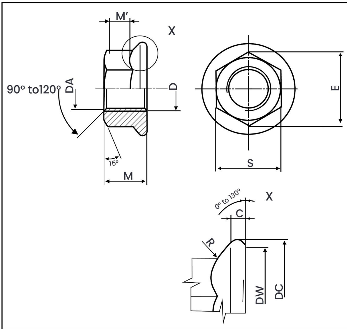
Metric Dimensions – DIN 6923 Hexagon Flange Nut
