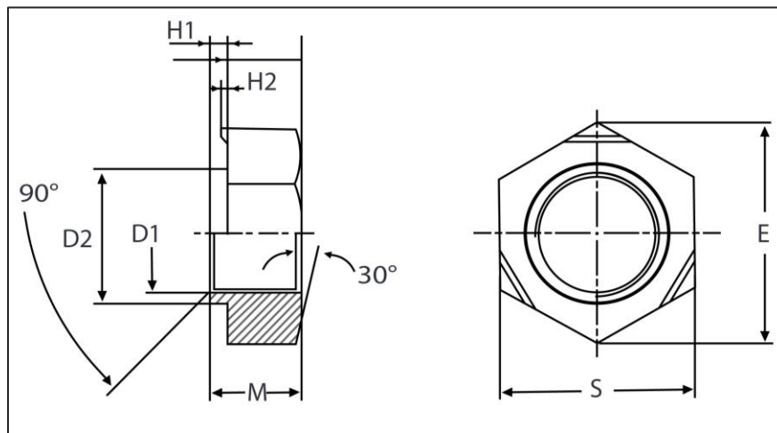
Metric Dimensions – DIN 929 Hexagon Weld Nut
