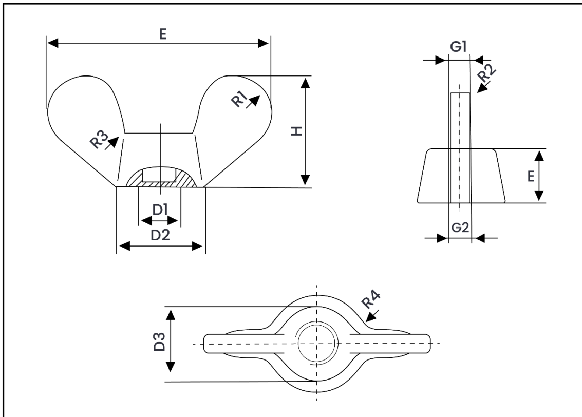
Weight Chart – DIN 315 Wing Nut
