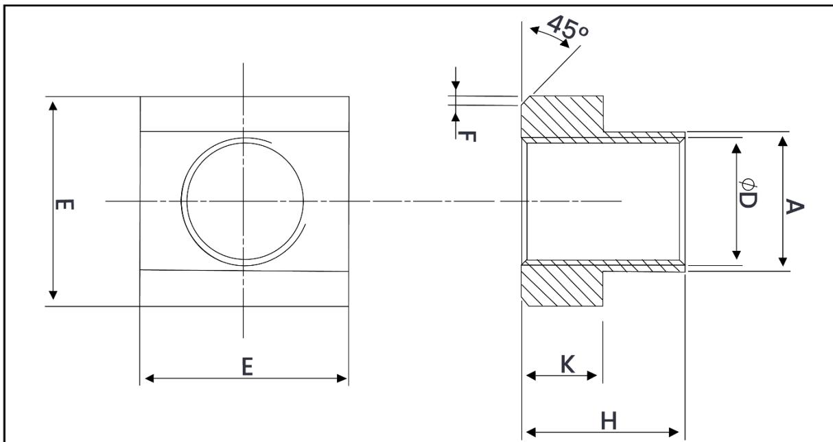
Weight Chart – DIN 508 T-Slot Nut
