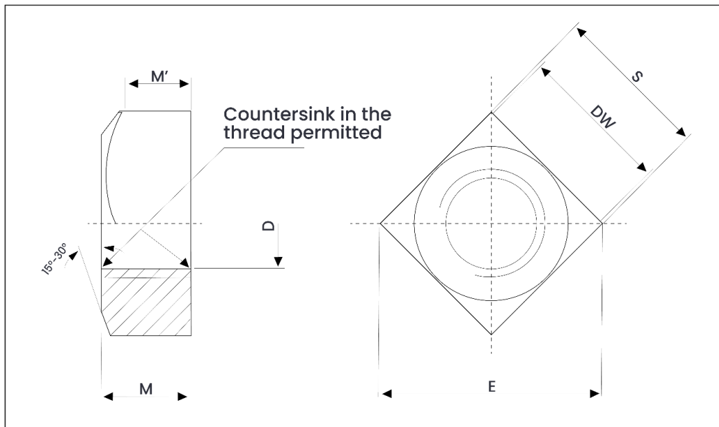
Weight Chart – DIN 557 Square Nut
