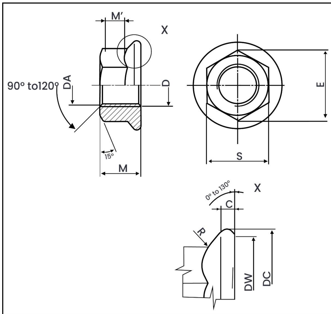
Weight Chart – DIN 6923 Hexagon Flange Nut
