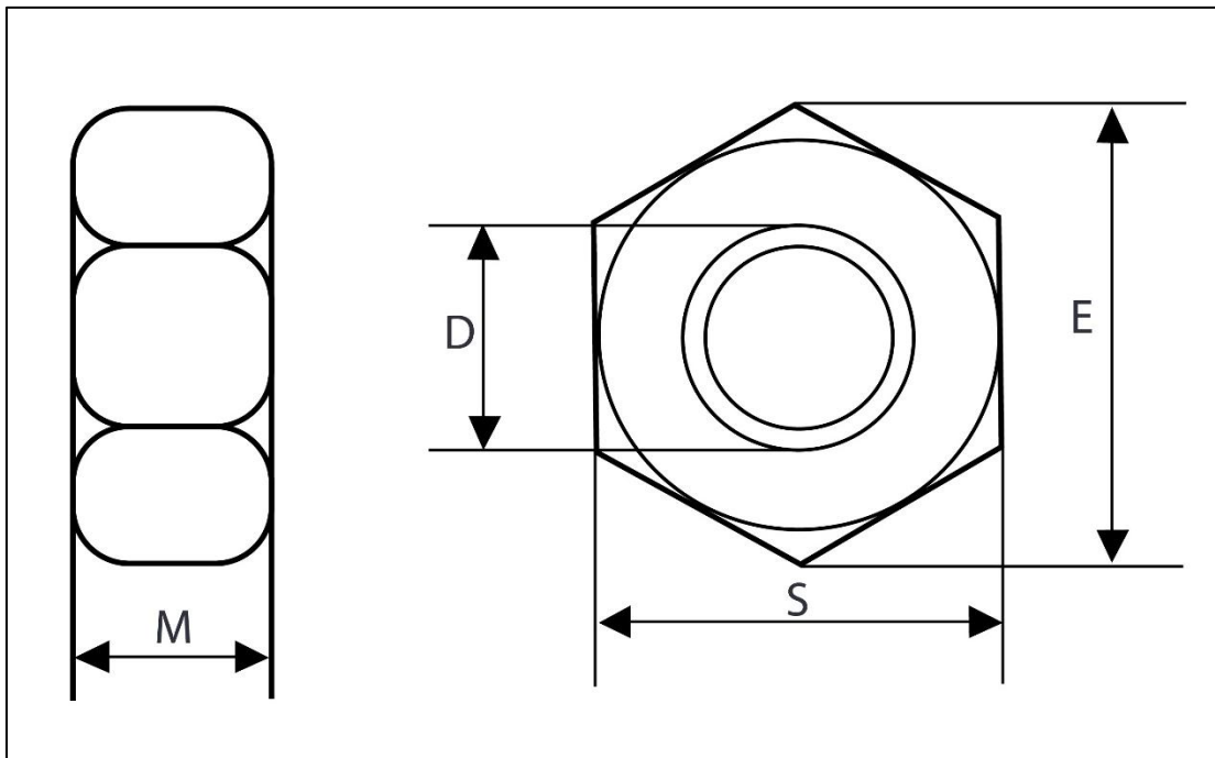
Weight Chart – DIN 934 Hexagon Nut
