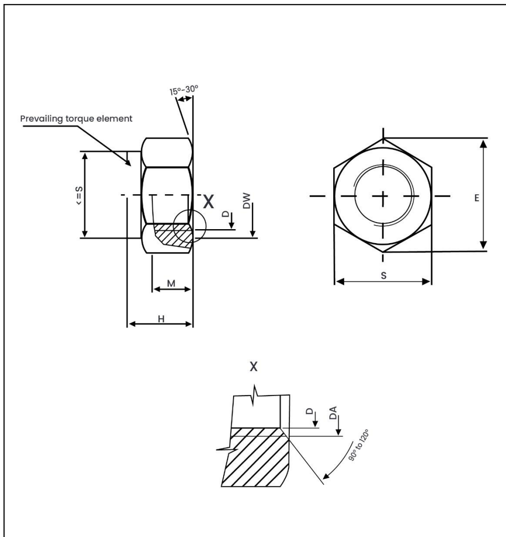
Weight Chart – DIN 980 All-Metal Hex Lock Nut
